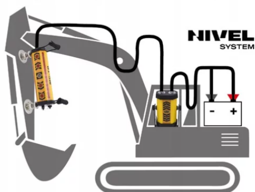
Schemat podłączenia z zasilaniem zewnętrznym
