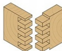
Połączenie wielowpustowe
